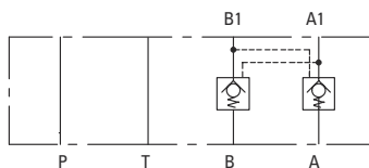
DGMPC-3-(D)AB*-(D)BA*
