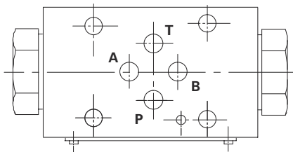
DGMPC-3-(D)AB*-(D)BA*-41
