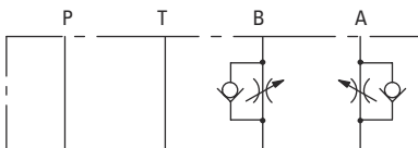
DGMFN-3-Z-P**
