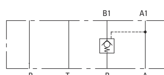
DGMPC-3-(D)BA*
