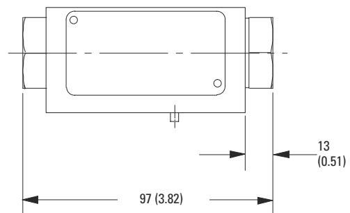
DGMPC-3-(D)BA*-41
