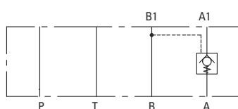
DGMPC-3-(D)AB*
