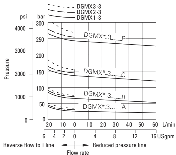
DGMX*-3-P*
