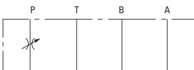
DGMFN-3-Z-P**
