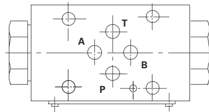
DGMPC-3-(D)AB*-41
