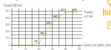
Progresividad del caudal en función de la carrera del gatillo
