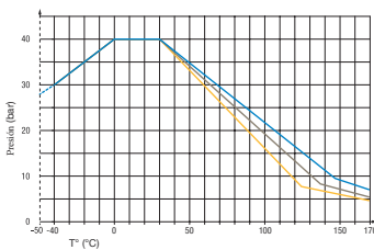
Presión - Temperatura
