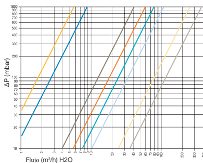
Pérdidas de carga
